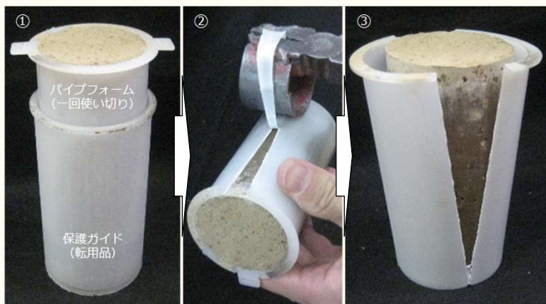
① 二重管構造のモールド缶
